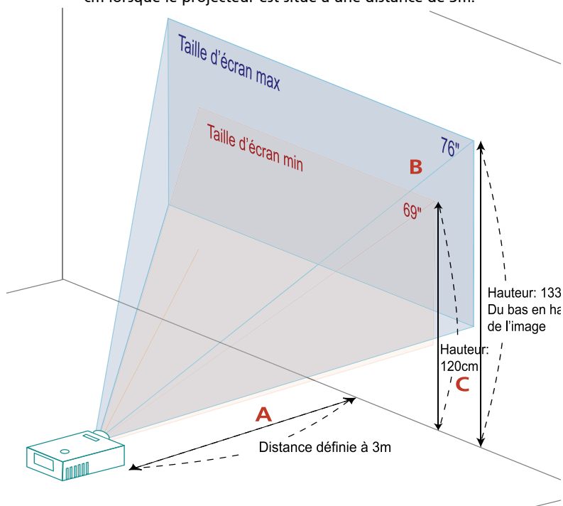
Figure: Distance fixe avec différents zooms et tailles d'écran. (Uniquement pour la série X1260, la série X1160 a un objectif à zoon fixe)
